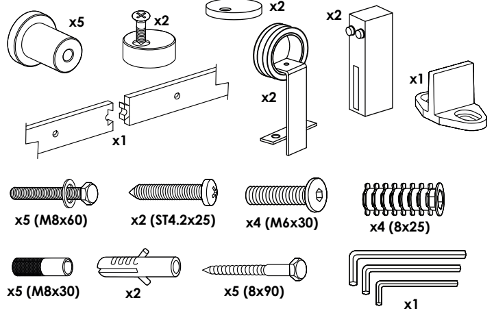
1B Montage op houten muur - Wand aus Holz Wooden wall - Mur à bois
