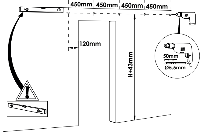
2B Montage op houten muur - Wand aus Holz Wooden wall - Mur à bois
