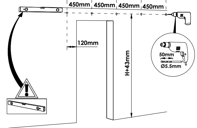
2B Montage op muur van steen/beton - Wand aus Stein/beton Stone/concrete wall - Mur à brique/béton
